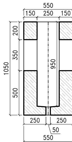
VELKÝ STOŽÁROVÝ ZÁKLAD 550/550/1050 mm
