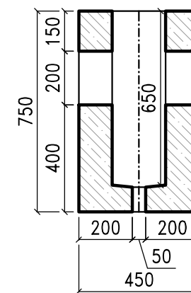
MALÝ STOŽÁROVÝ ZÁKLAD 450/450/750 mm
