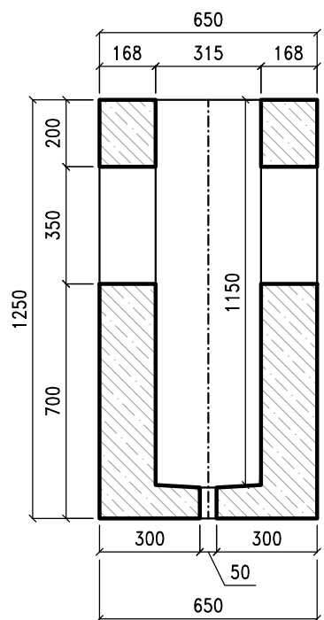
VELMI VELKÝ STOŽÁROVÝ ZÁKLAD 650/650/1250 mm
